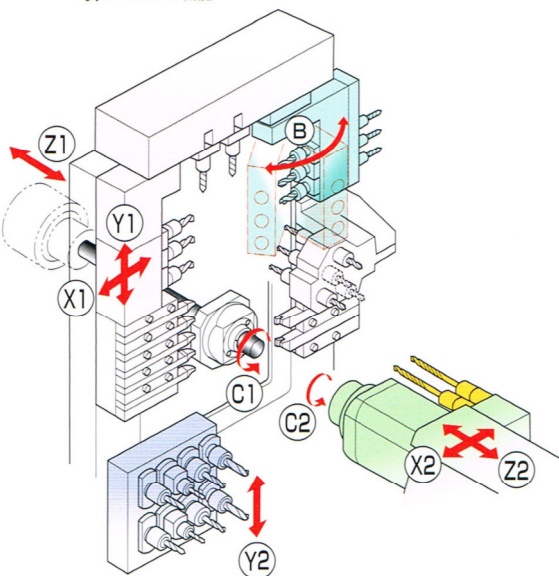
刃物台イラスト：タイプB
